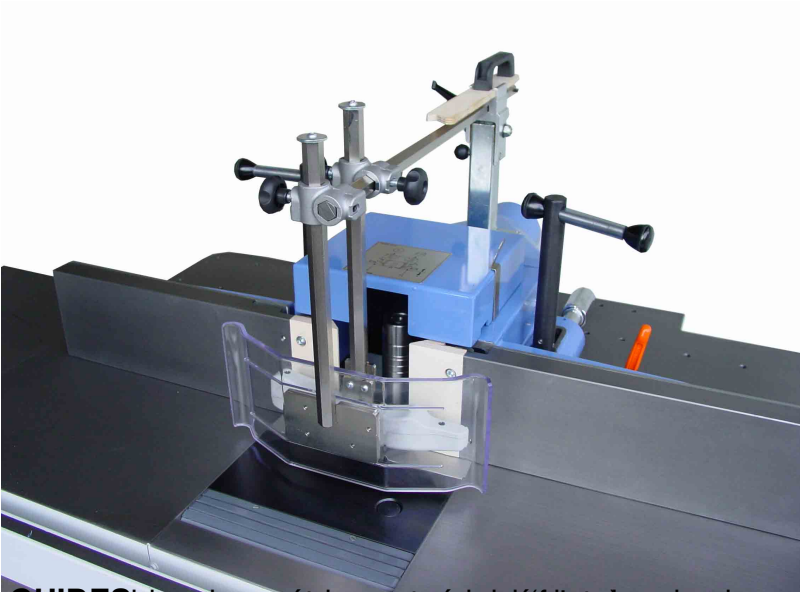
GUIDES Side micrométrique standard / frottoir de plaques de sécurité en fonte avec lèbres interchangeables
